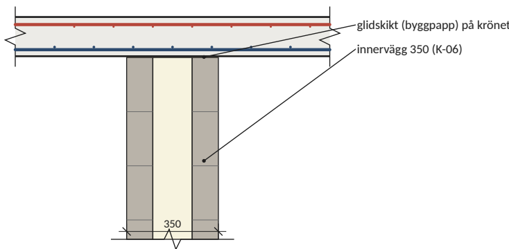
SEKTION D-D Innervägg (V15)
