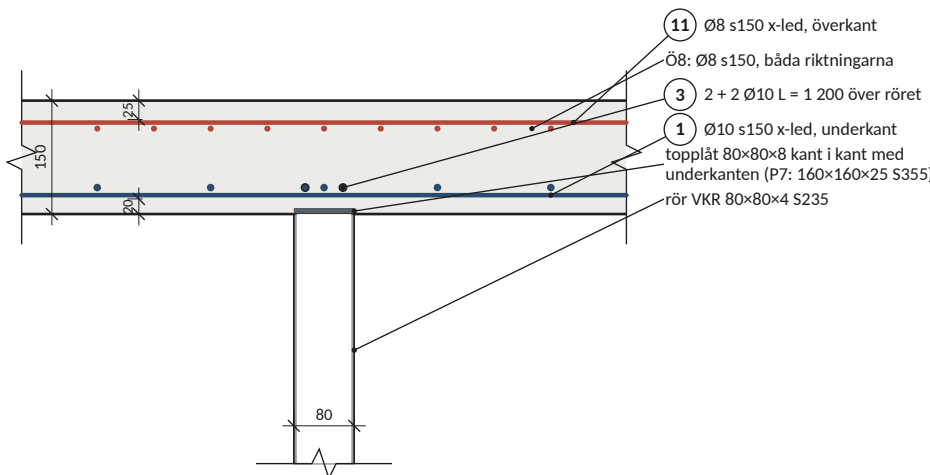
SEKTION B-B Vid rör (P5)
