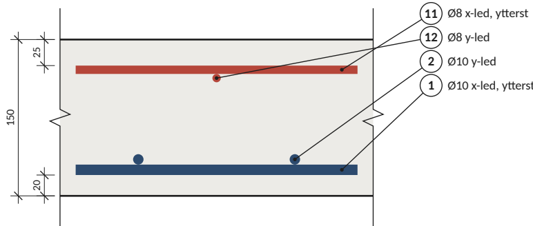
DETALJ F Armeringens lägen
