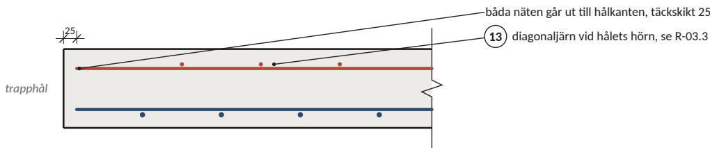
SEKTION C-C Trapphålets kant
