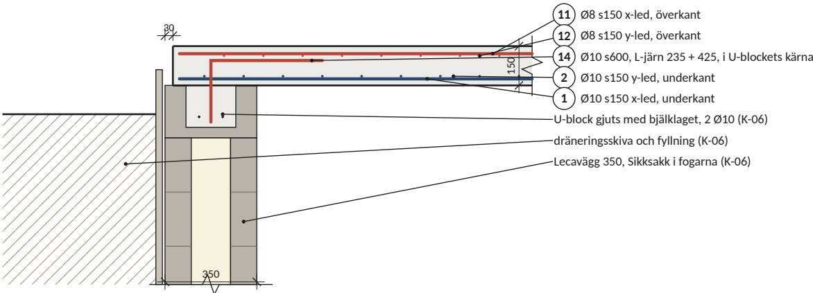
SEKTION A-A Yttervägg mot jord (V14)
